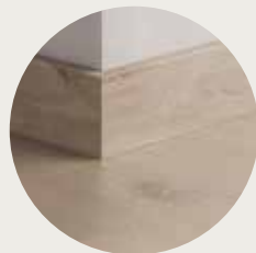
DOPASOWANA KOLORYSTYCZNIE LISTWA PRZYPODŁOGOWA PARKIETOWA 2400 × 14 × 77 mm PGPSK(-)
